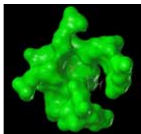
SBDD & FBDD
